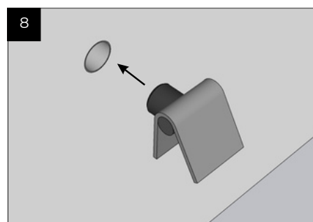
Encaixar o balizador na parede
