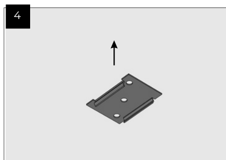
Posicionar a mola de fixação no local marcado de acordo com projeto
