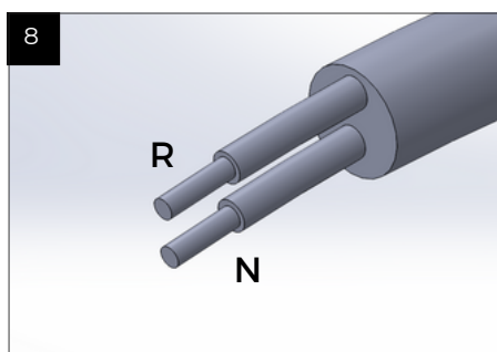
Ligar retorno e neutro do driver com a alimentação elétrica conforme a imagem
