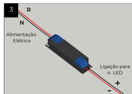
Driver em local remoto
