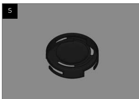
Posicionar a tampa de fixação no local marcado de acordo com projeto
